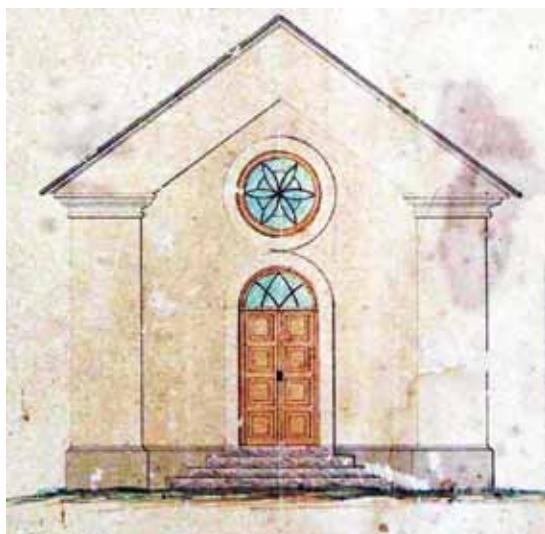
Capela católica na Colônia de Santa Isabel – Desenho do engenheiro Albert Jahn – janeiro de 1861. ACERVO: ARQUIVO PÚBLICO DO ESTADO DO ESPÍRITO SANTO
